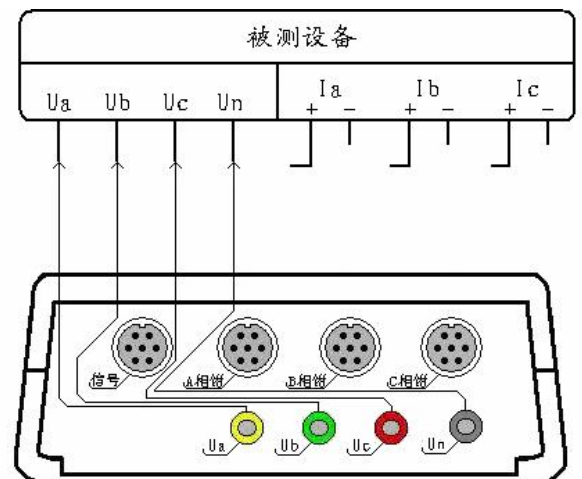
电压谐波测试接线图
